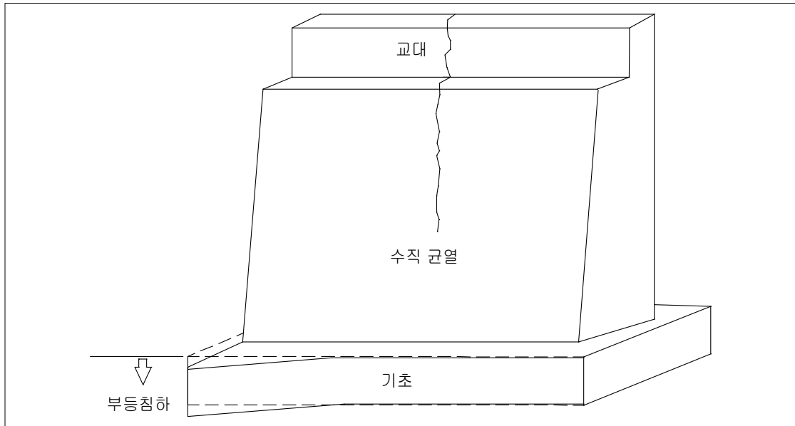
【그림 3.2.8】 부등침하로 인한 교대의 수직균열
